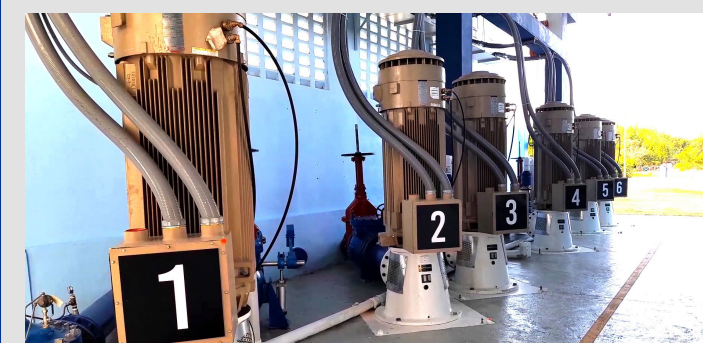
Rehabilitación de la obra de toma del contraembalse de López
